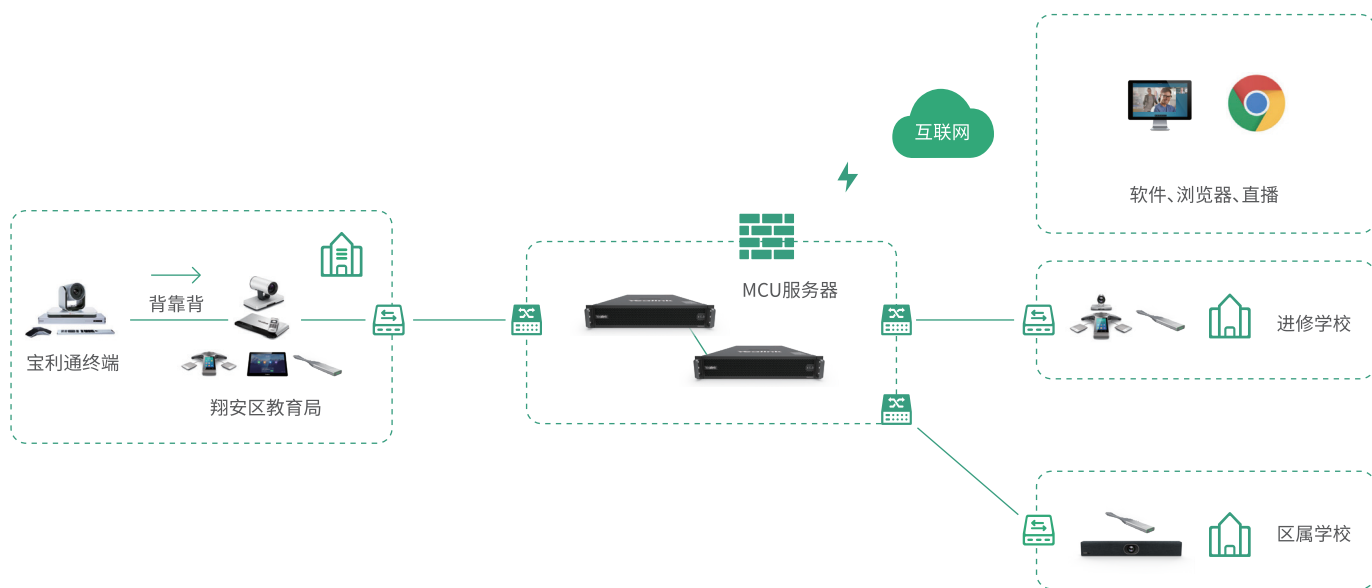
方案组网图
