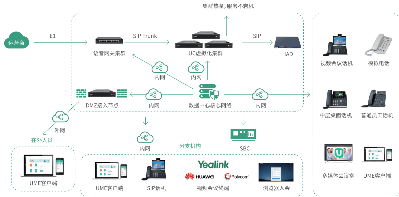
方案组网图
