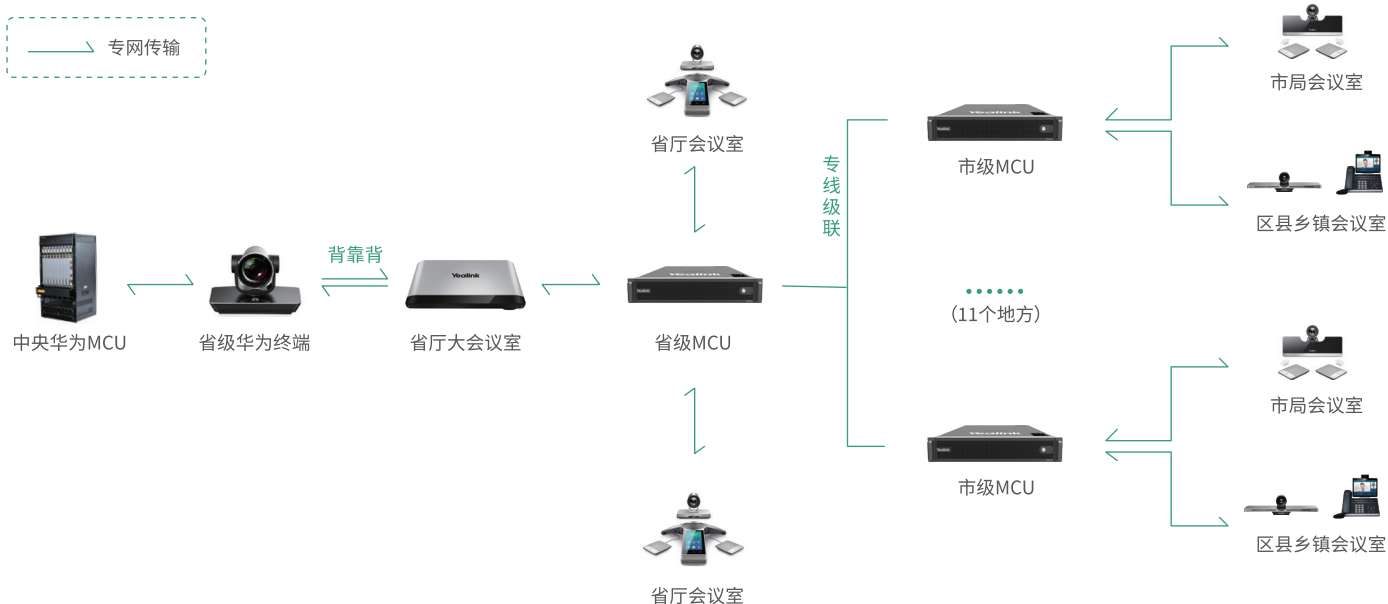
方案组网图
