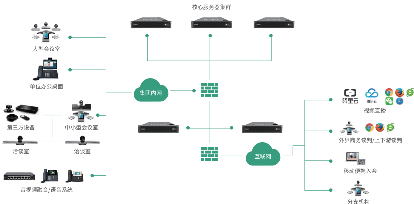
方案组网图
